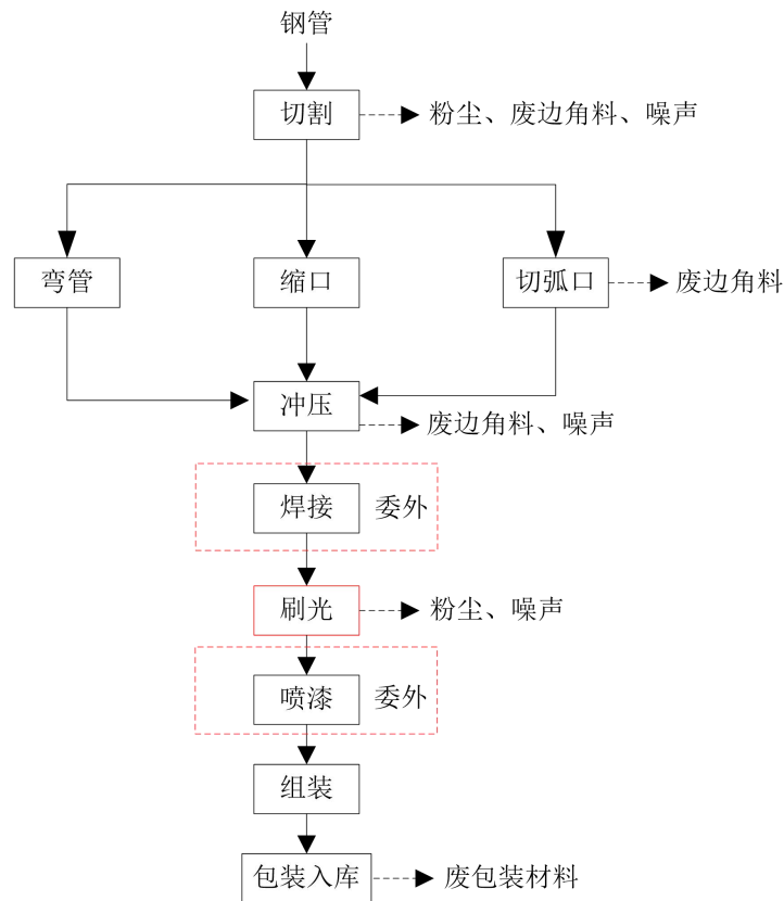
图 2-2 生产工艺流程及产污环节图
