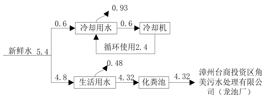
图 2-1 项目水平衡图 (单位: t/d)
