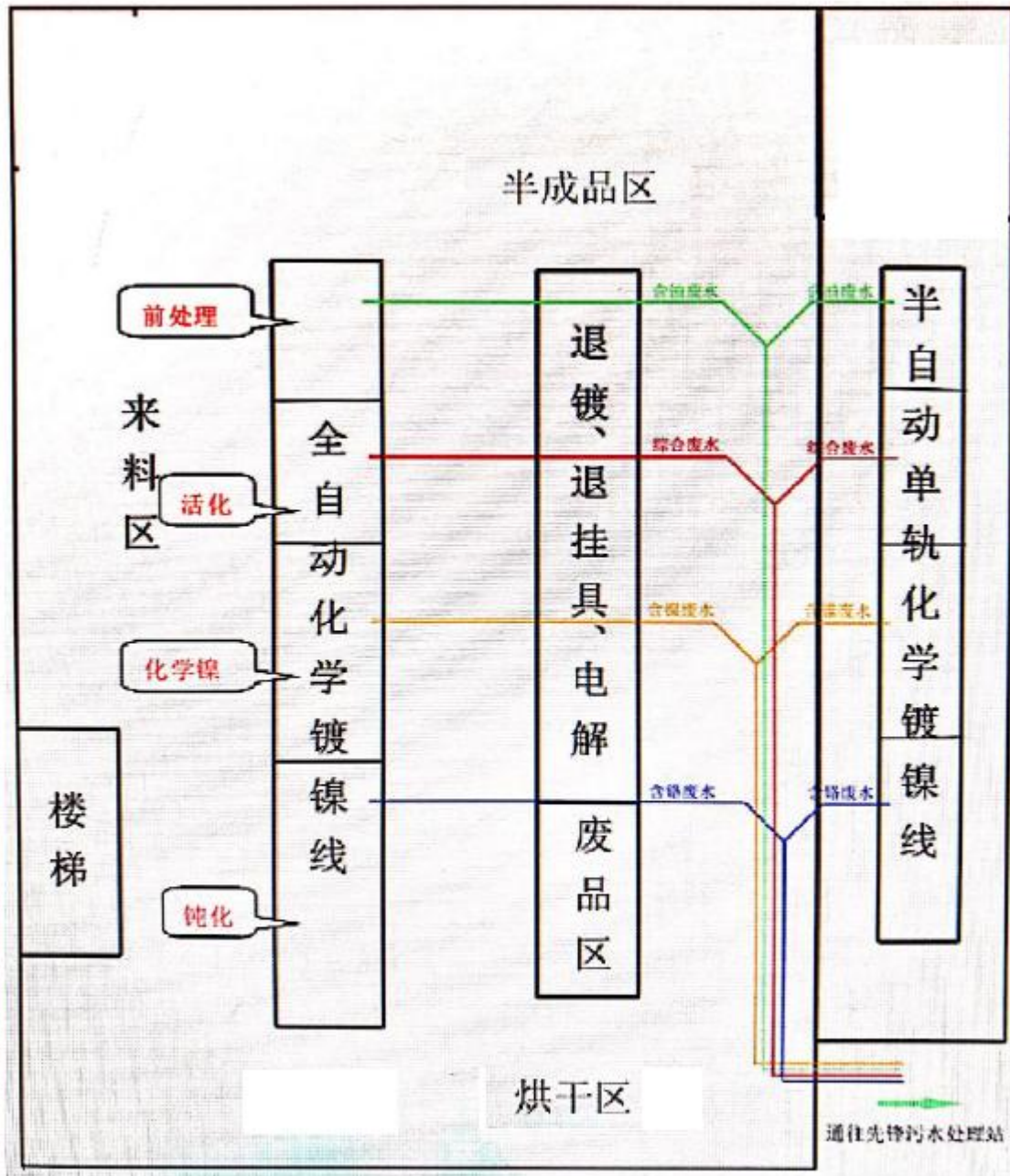
欣鑫瑞生产废水分质分流图
