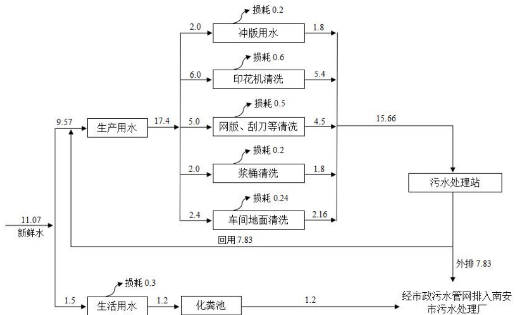
图 2-1 水平衡 单位：m 3 /d
