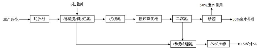
图 4-1 生产废水处理工艺流程图
