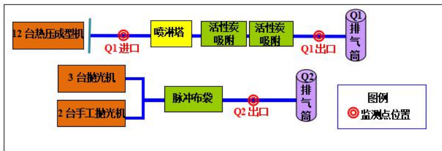
图4-3 项目废气处理工艺流程图
