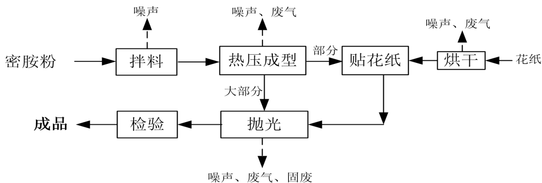
图 3-2 生产工艺流程及污染物产生环节
