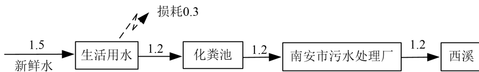
图 3-1 项目水平衡图 (m 3 /d)
