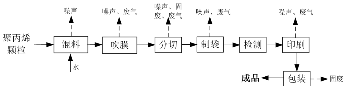
图 3-2 生产工艺流程及污染物产生环节
