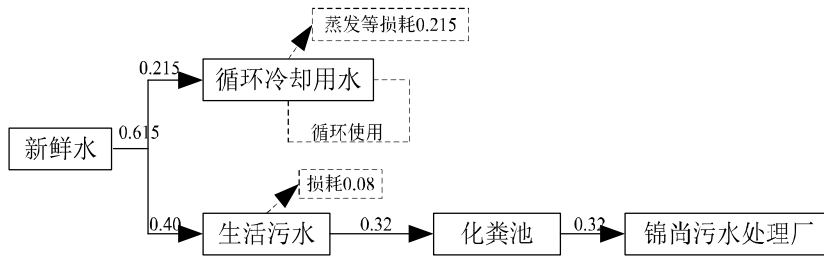
图3-1 项目水平衡图（单位：t/d）
