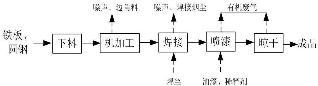
图 4-2 轮毂生产工艺流程及污染物产生环节
