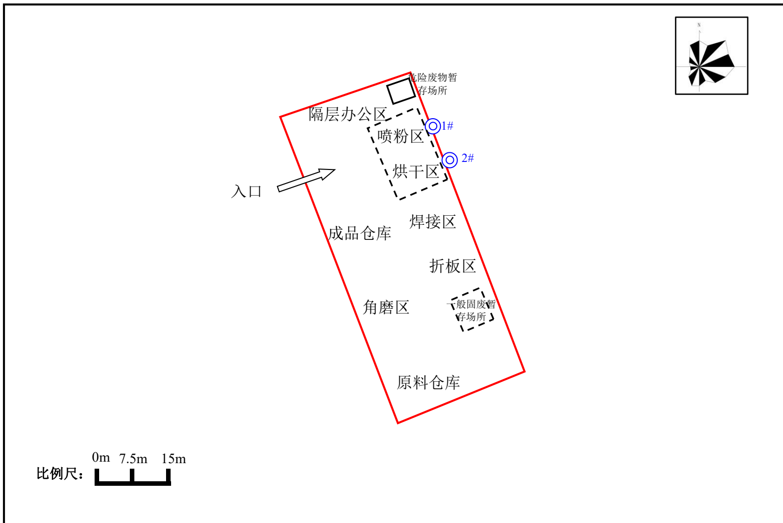
附图 6 项目车间平面布置图
