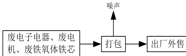
图 2.8-3 废电子电器、废电机、废铁氧体铁芯回收仓储工艺流程及产排污图
