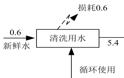
图 2.7-1 项目水平衡图（单位：t/d）
