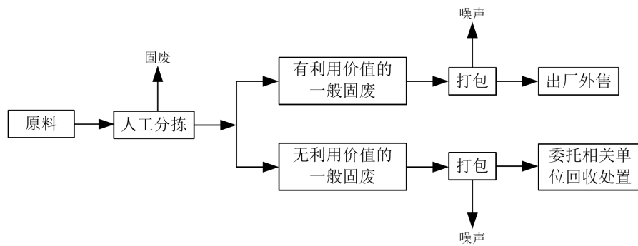
图 2.8-2 一般固废（可回收）加工处理工艺流程及产排污图
