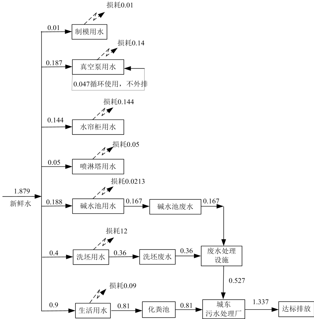
图 3-1 项目水平衡图 (单位: t/d)
