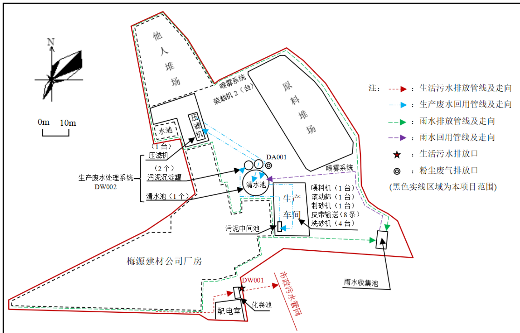
附图3 项目厂区布置示意图
