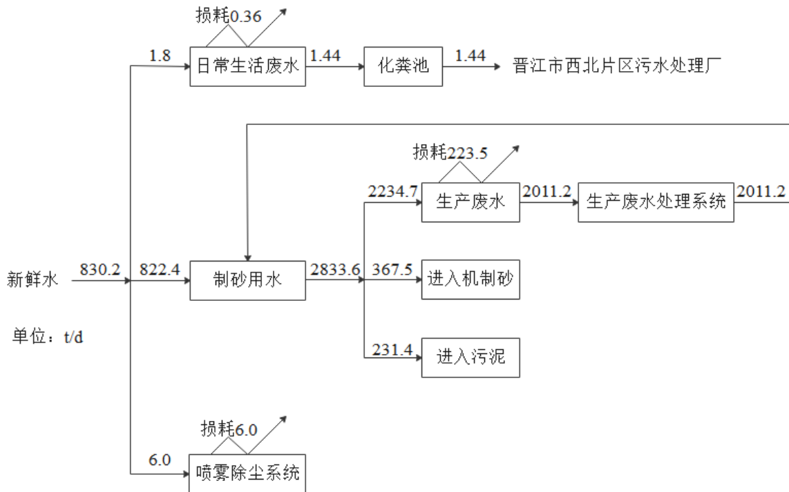
图 3-2 项目供排水平衡图
