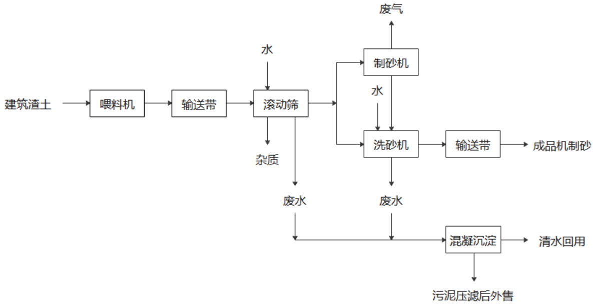
图 3-1 工艺流程图
