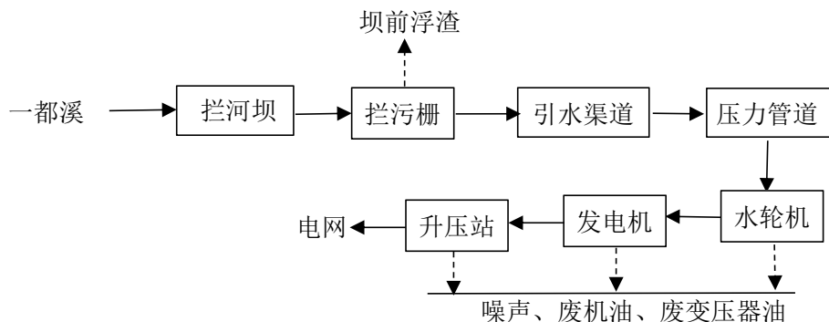
图 2-1 工程运行方式图
