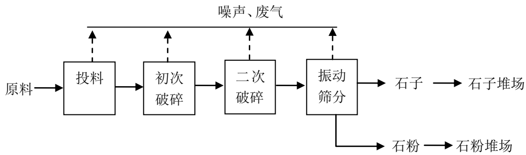
图 3-2 项目生产工艺流程图
