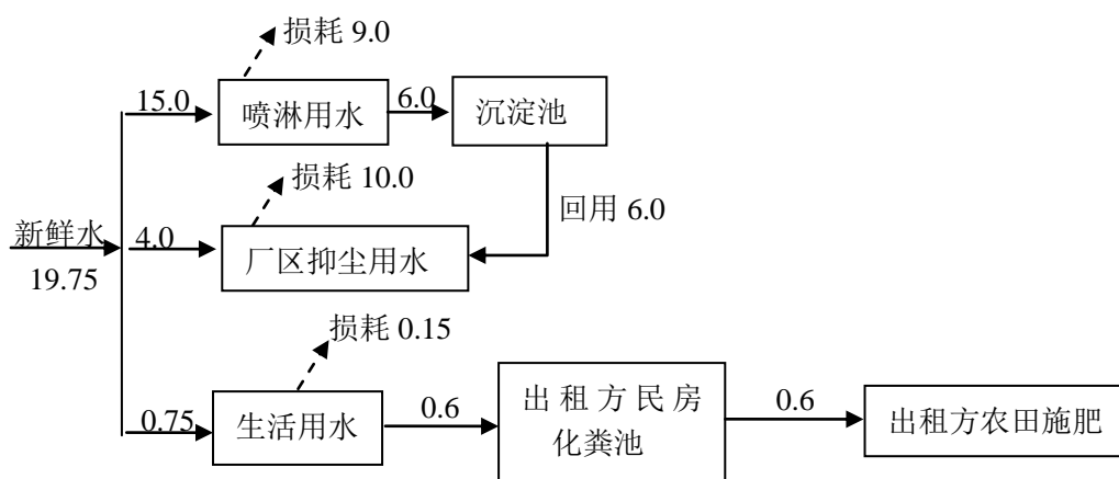
图 3-1 项目水平衡图(单位: \text{m}^3/\text{d} )
