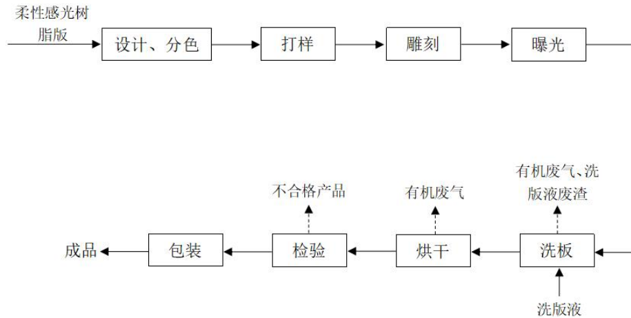
图 2-2 柔性印刷版生产工艺及产污环节图
