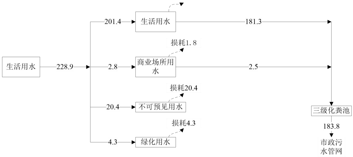
图 3-4 项目用排水水平衡图
