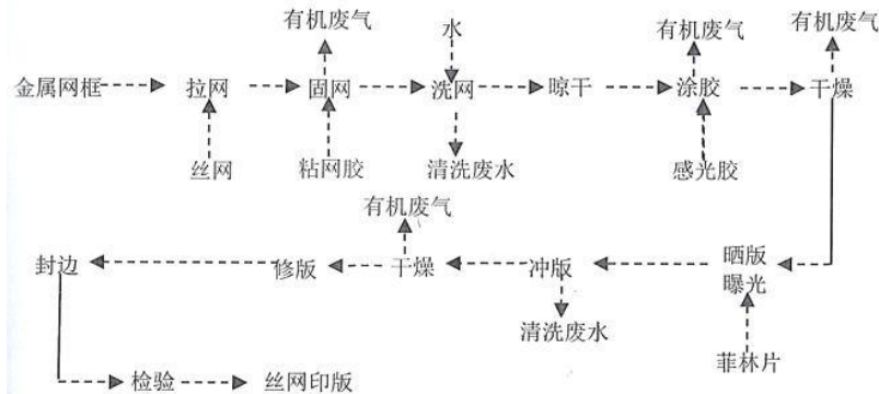
图 3-3 制版生产工艺流程图
