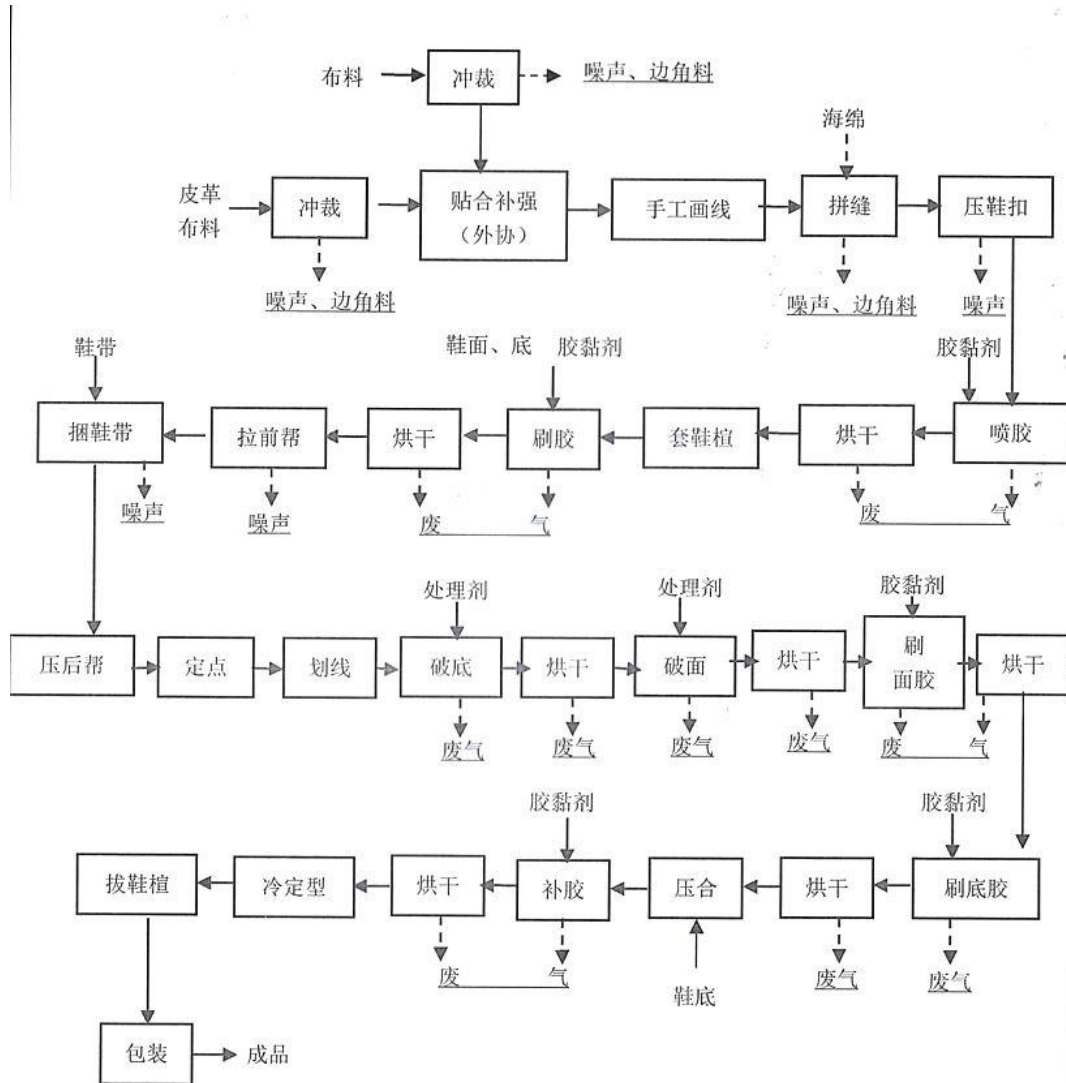
图 3-6 制鞋生产工艺流程图
