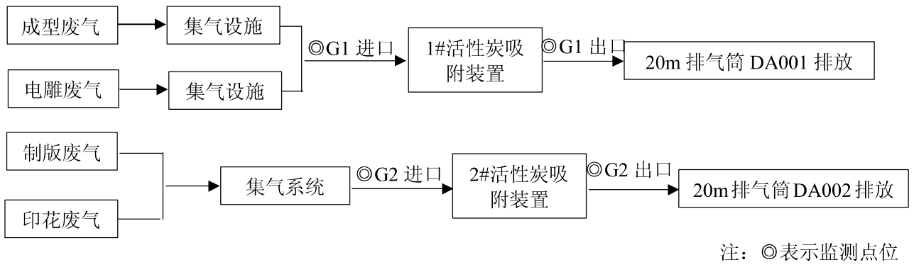
图 4-3 废气处理工艺流程图
