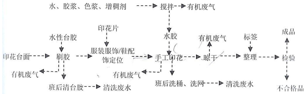
图 3-4 印花台面印花生产工艺流程图
