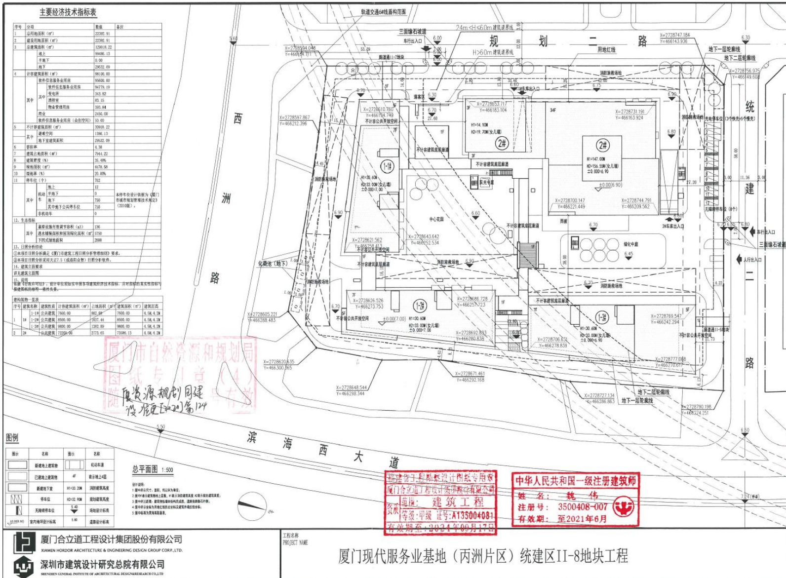
图 3-4 项目平面布置图
