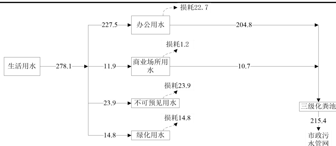
图 3-4 项目用排水水平衡图
