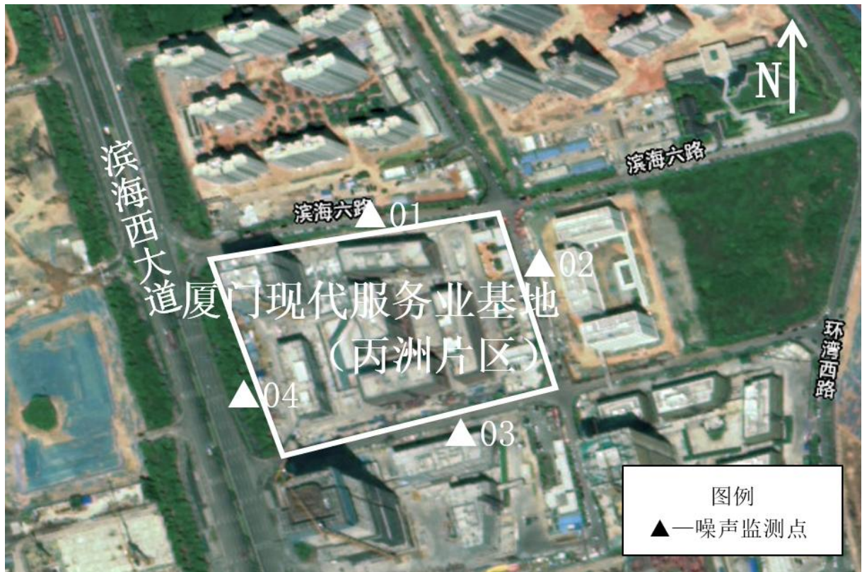
图 7-1 边界噪声监测点位图
