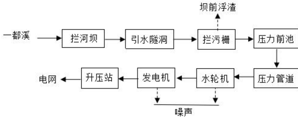
图 3-1 工程运行方式示意图
