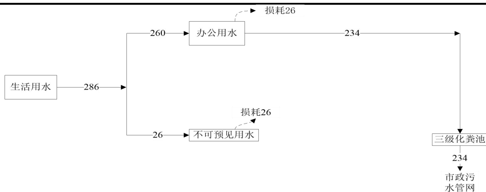
图 3-5 项目用排水水平衡图
