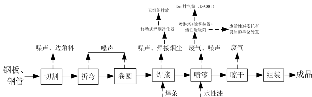
图 3-2 链条生产工艺流程及污染物产生环节
