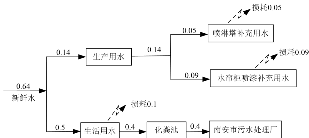
图 3-1 项目水平衡图 (m³/d)
