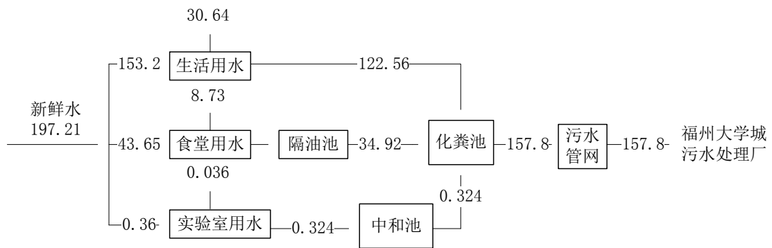
图 4.2-1 项目水平衡图 (t/d)
