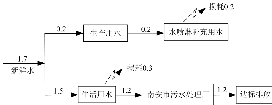
图 2-1 项目水平衡图（单位：t/d）
