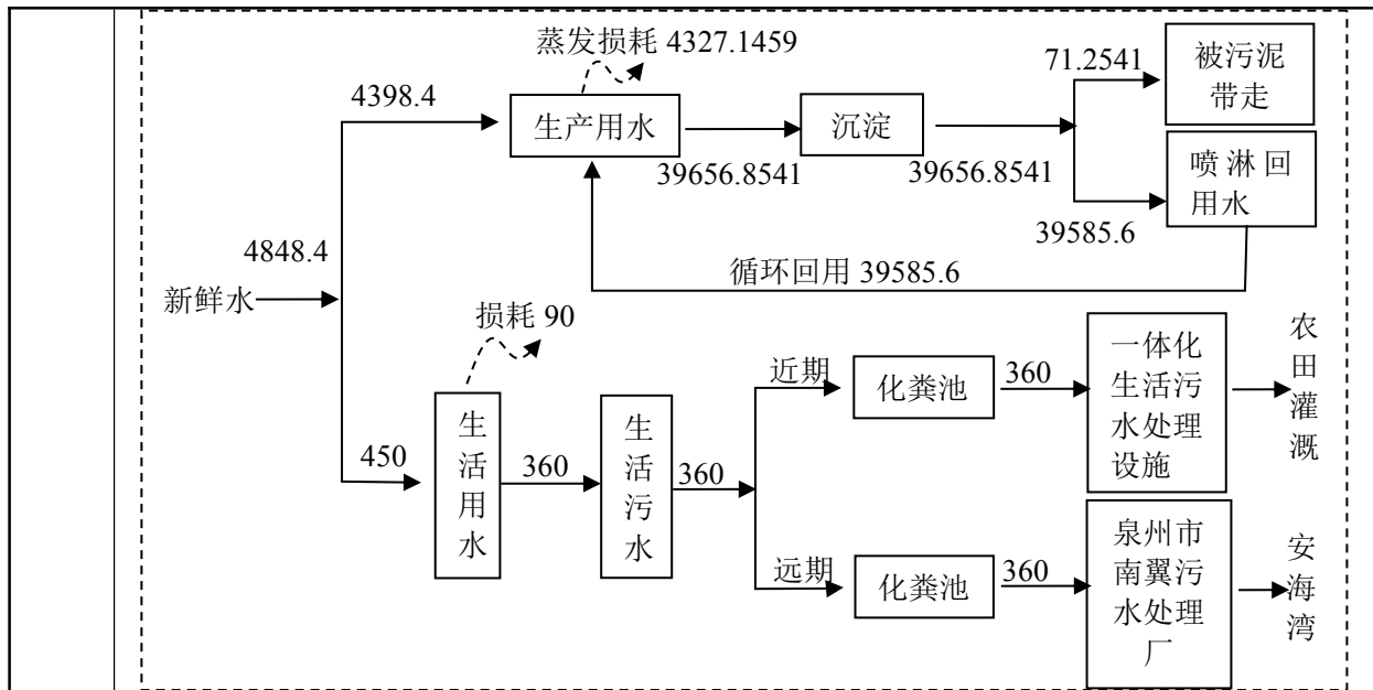
图 2-2 扩建后项目水平衡图 (单位: m 3 /a)
