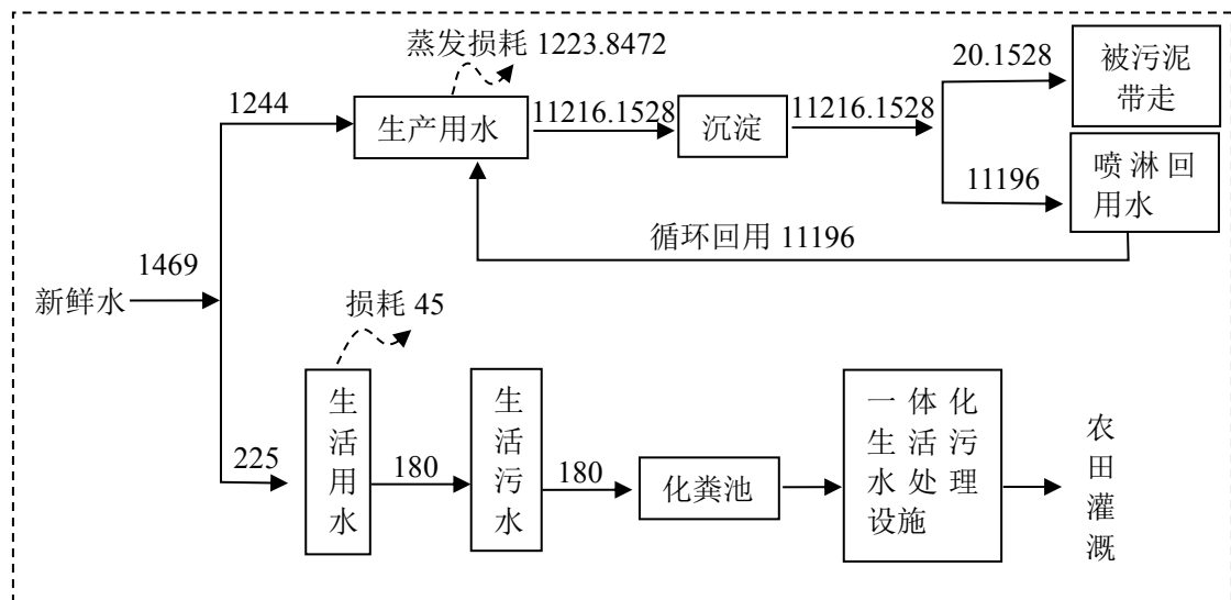
图 2-6 扩建前项目水平衡图 (单位: m 3 /a)
