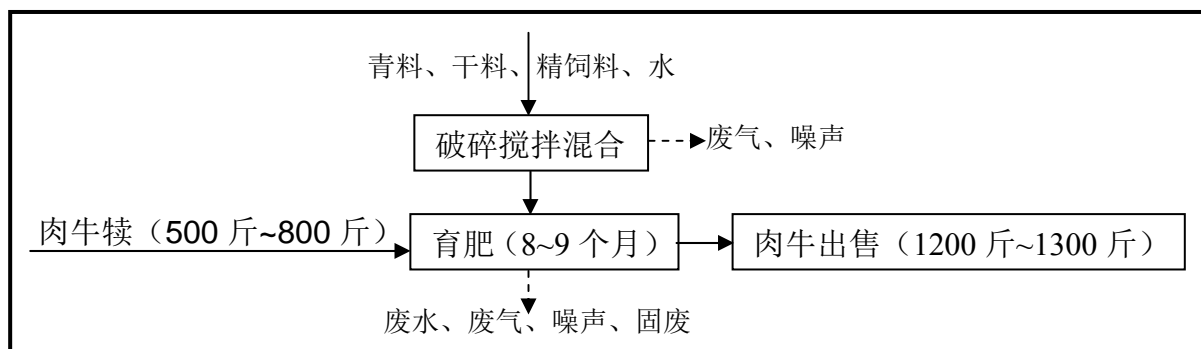
图 3.5-1 项目养殖工艺及产污环节流程图
