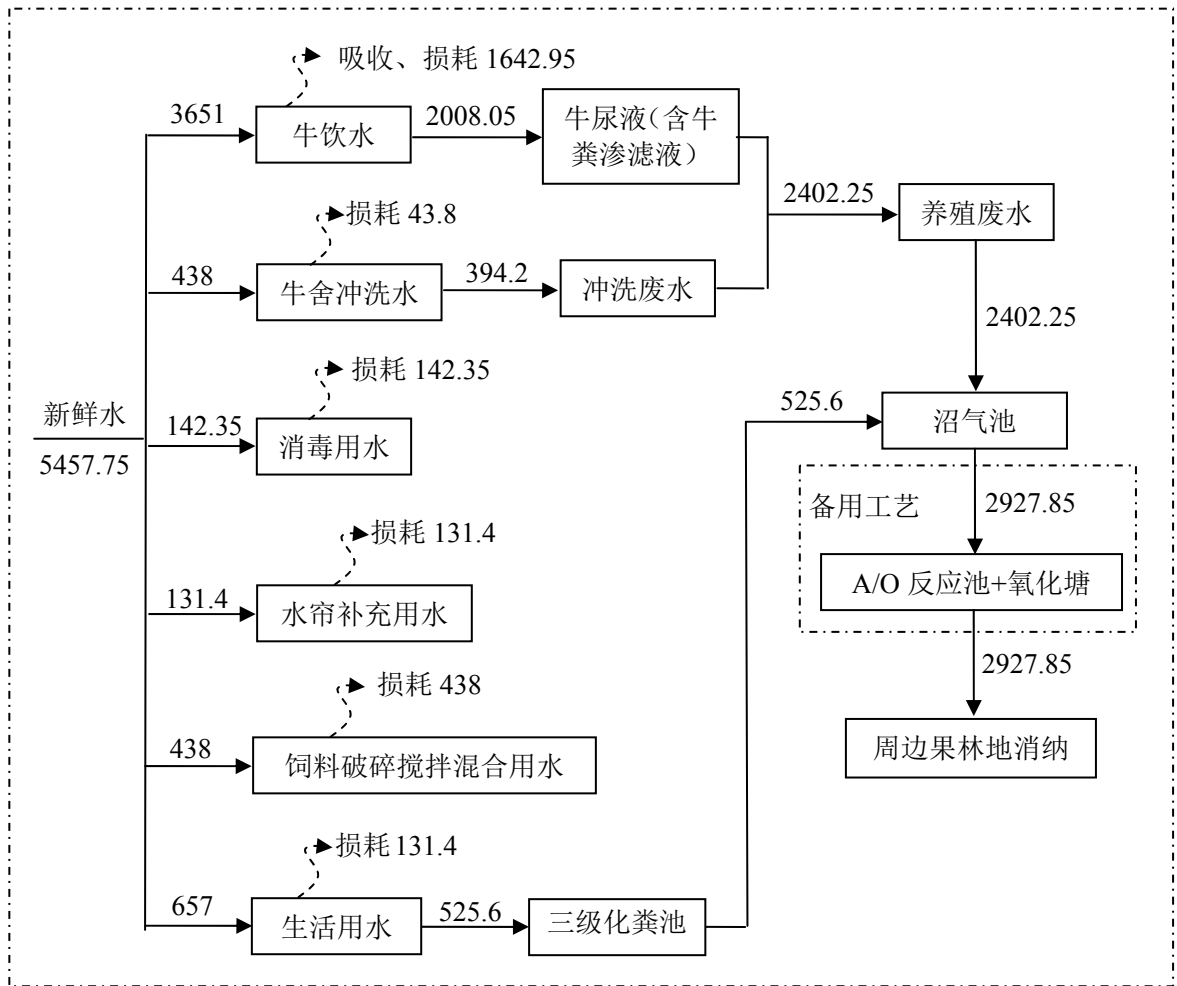
图 3.6-1 项目水平衡图 单位: t/a
