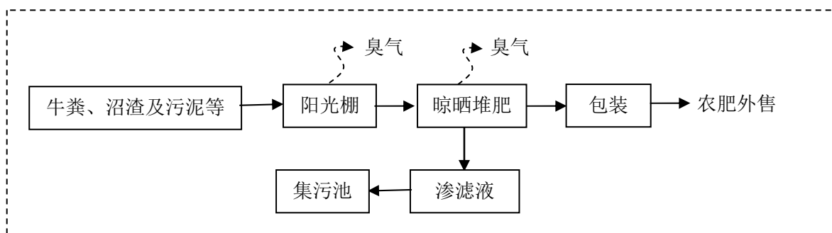
图 3.5-3 农肥加工工艺流程图
