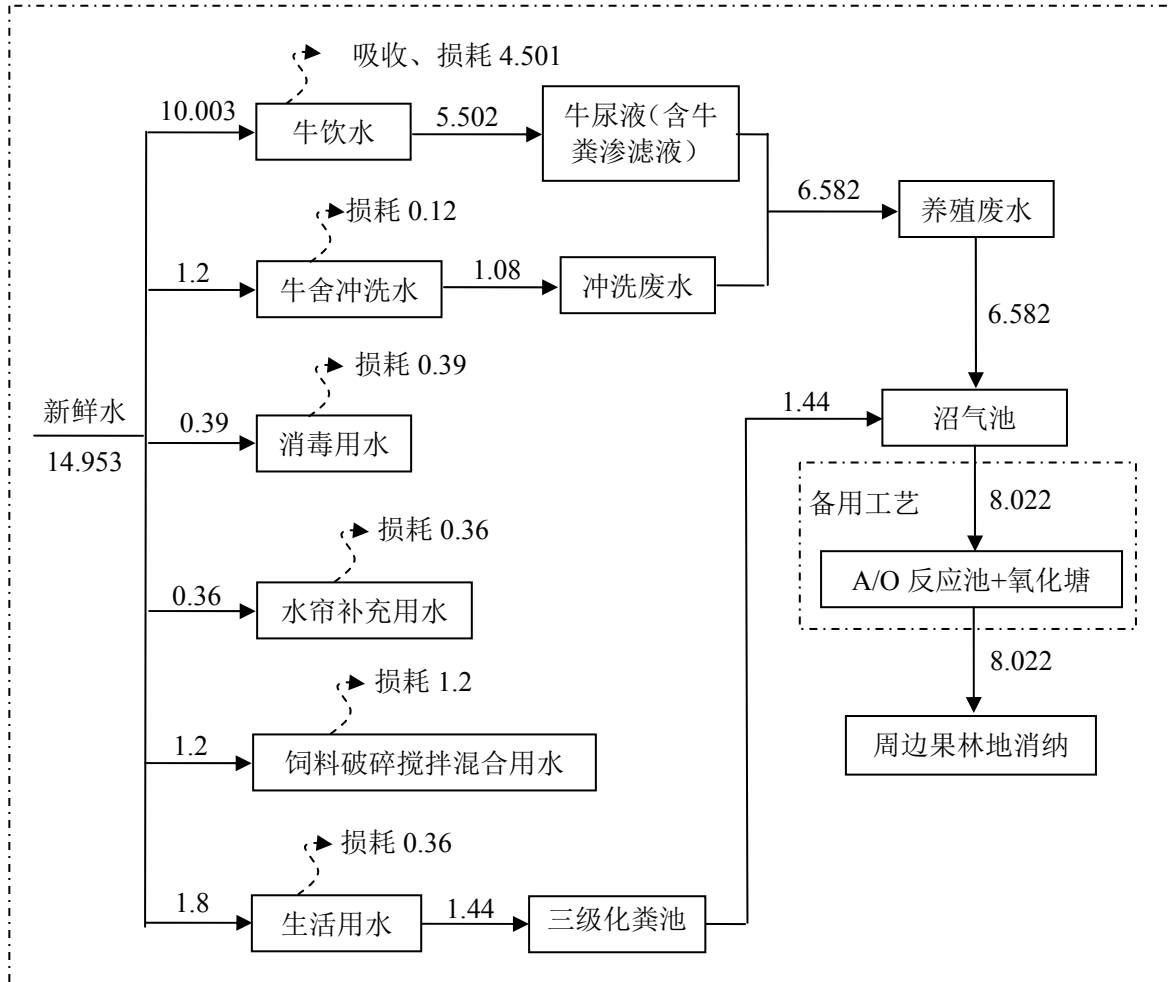
图 3.6-2 项目日均水平衡图 单位：t/d
