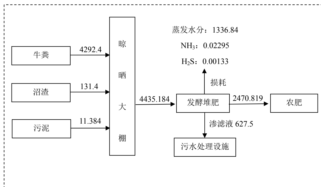
图 3.5-4 农肥物料平衡图
