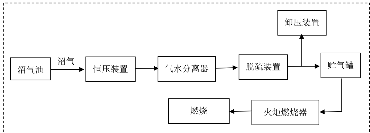
图 3.5-5 沼氣燃燒工藝流程圖
