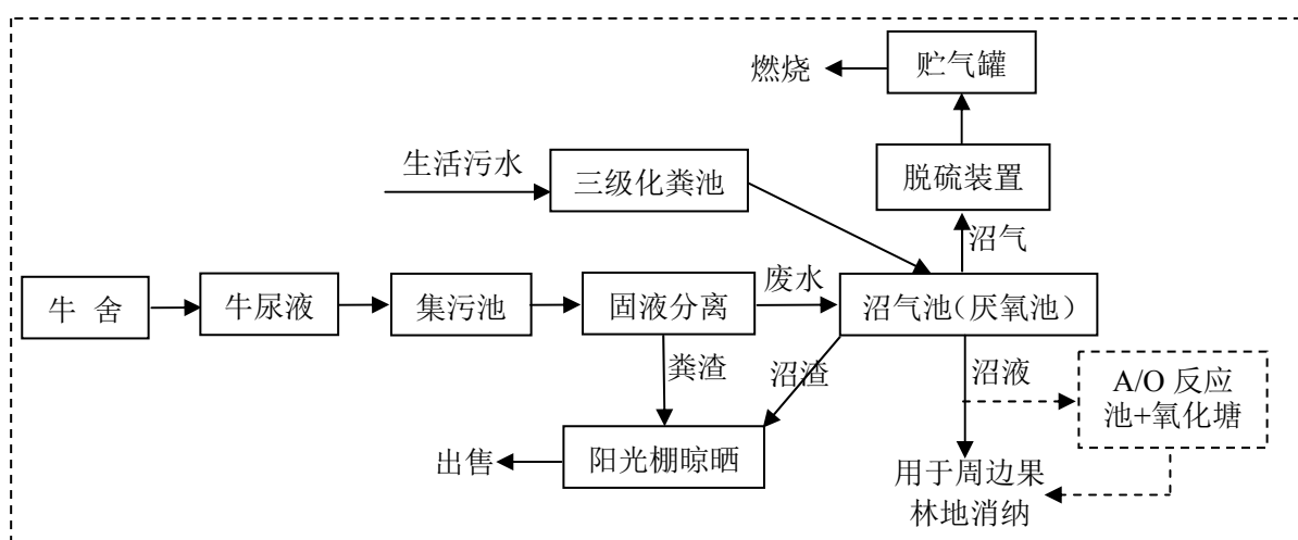
图 3.5-2 废水处理工艺流程图 (A/O 反应池+氧化塘为备用工艺)
