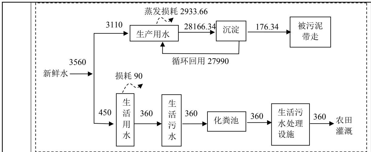
图 2-5 技改前项目水平衡图 (单位: \text{m}^3/\text{d} )
