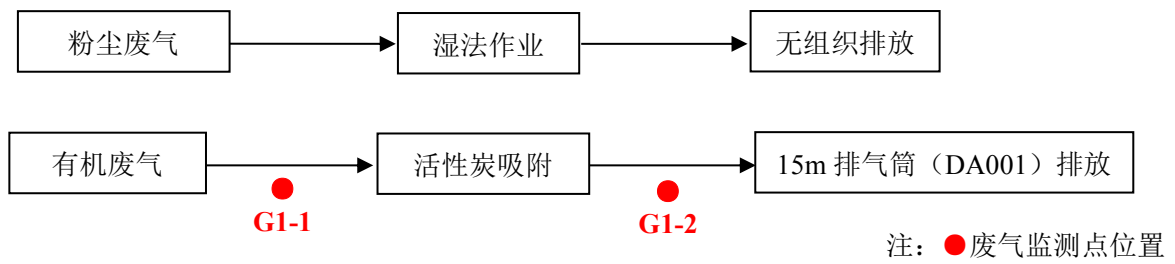
图 4-2 项目废气处理流程示意图
