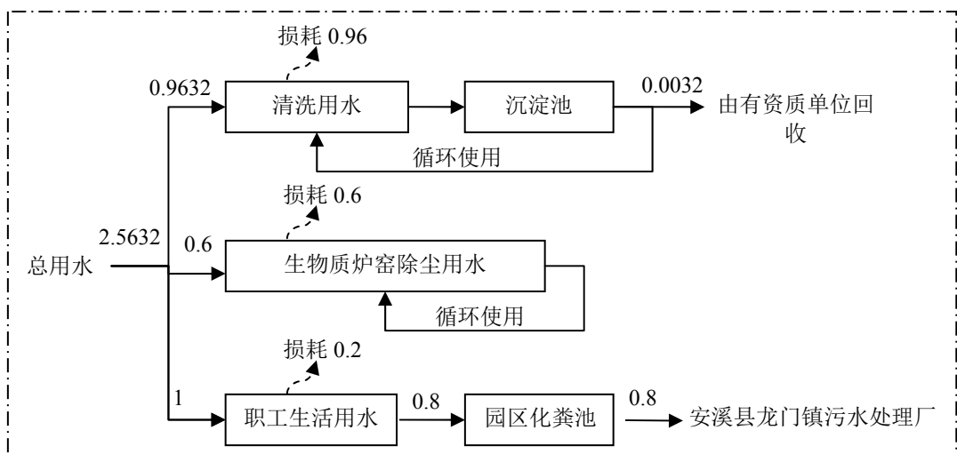
图 4.2-5 项目水平衡图 (单位 t/d)
