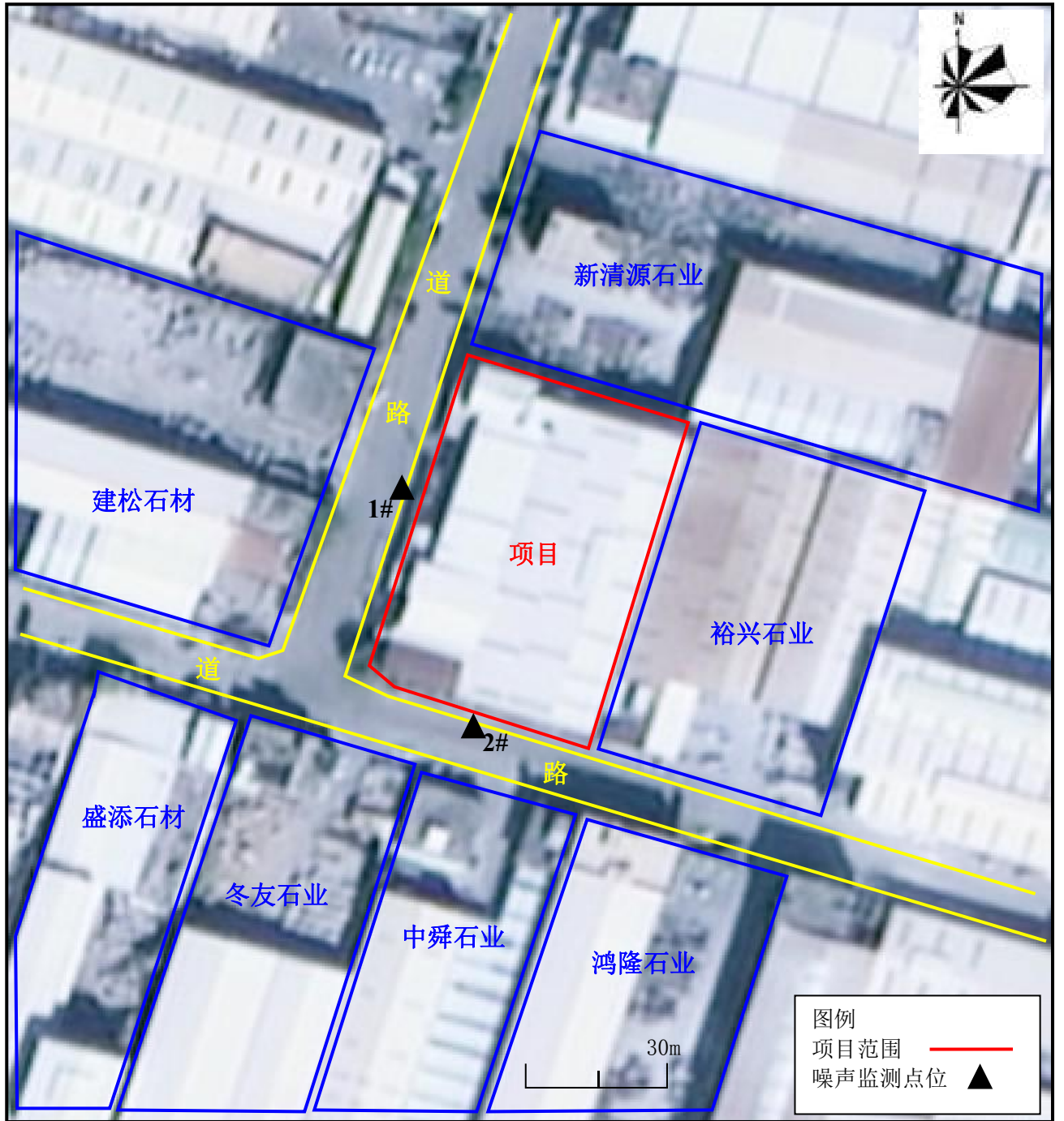
附图 2-1 项目周边环境示意图及监测点位图
