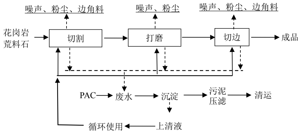
图 2-4 扩建前花岗岩石板材、异形石材生产工艺及产污环节示意图
