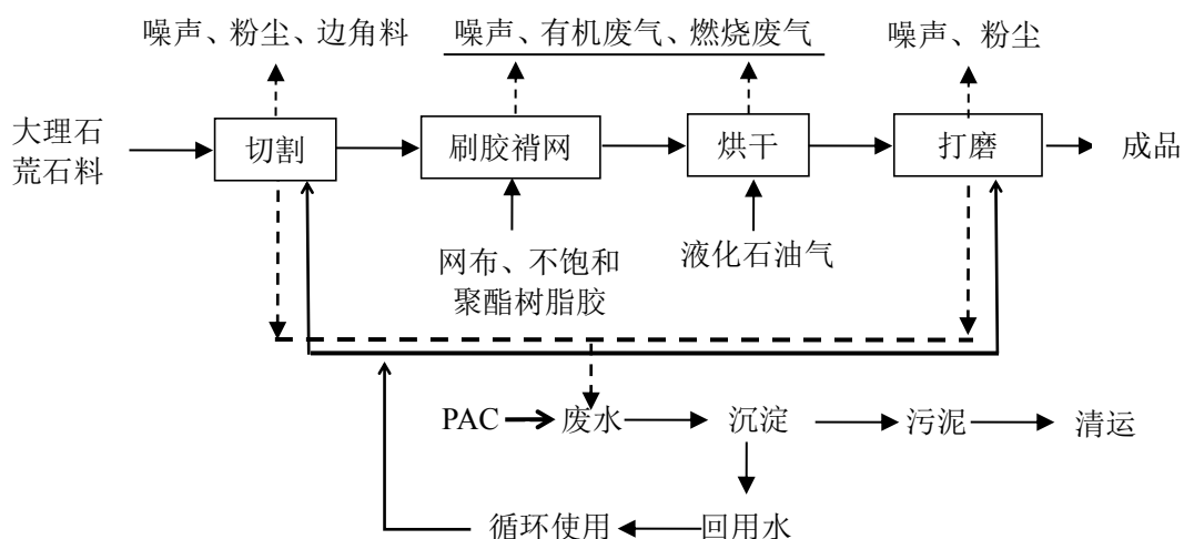
图 2-6 扩建后大理石材生产工艺及产污环节示意图
