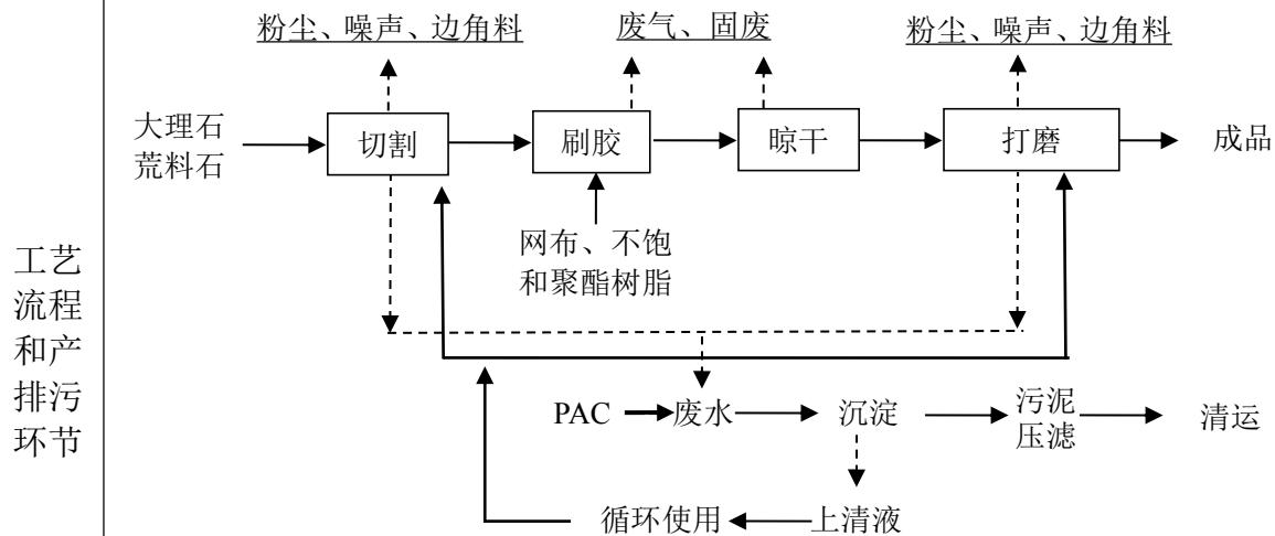
图 2-3 扩建前大理石板材生产工艺及产污环节示意图
