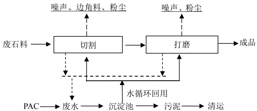
图 2-5 扩建前马赛克生产工艺及产污环节示意图
