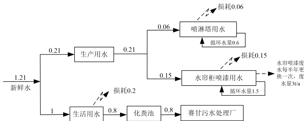
图 3-1 项目水平衡图 (m³/d)
