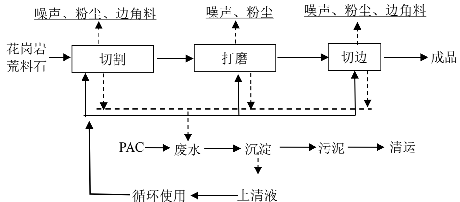
图 2-3 扩建前项目石板材生产工艺流程图
