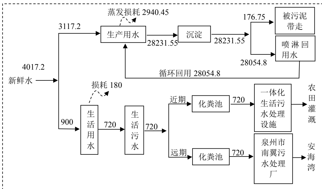
图 2-2 扩建后项目水平衡图 (单位: \text{m}^3/\text{a} )
