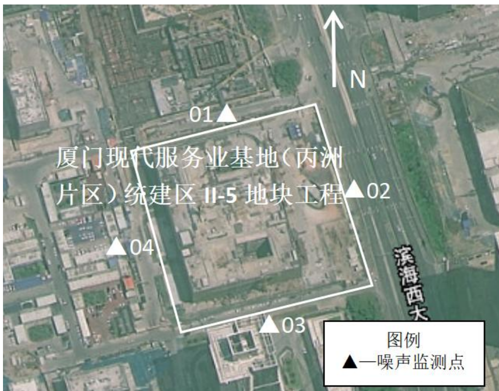
图 7-1 边界噪声监测点位图
