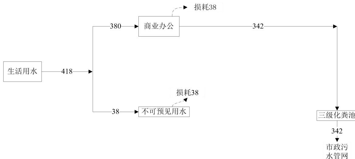
图 3-5 项目用排水水平衡图
