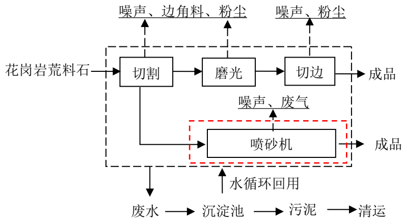
图 3-6 花岗岩板生产工艺及产污环节流程图
