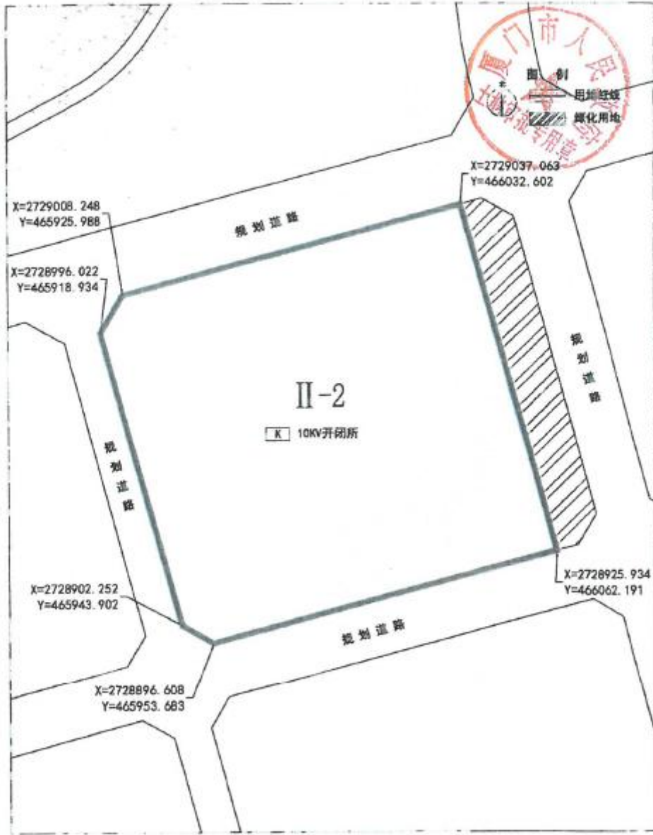
2015TG02 地块 II-2 子地块出让宗地平面界址图
