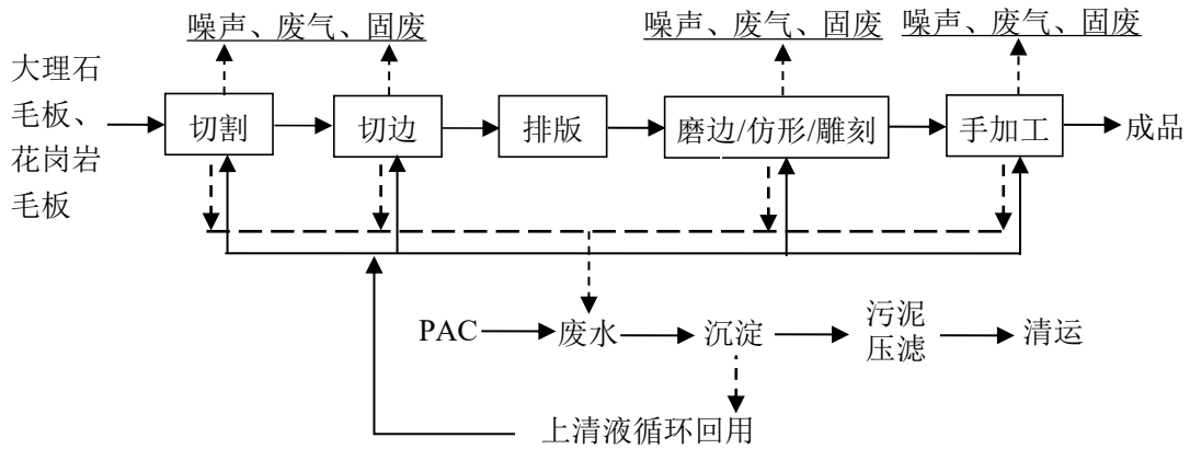
图 2-2 花岗岩石板材工艺流程及产污环节示意图
