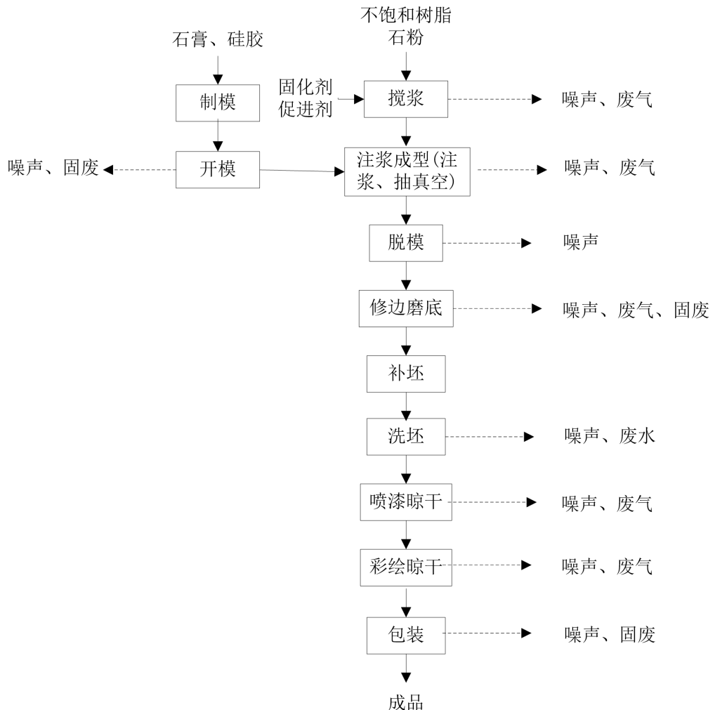
图 2-2 项目生产工艺及产污环节示意图
