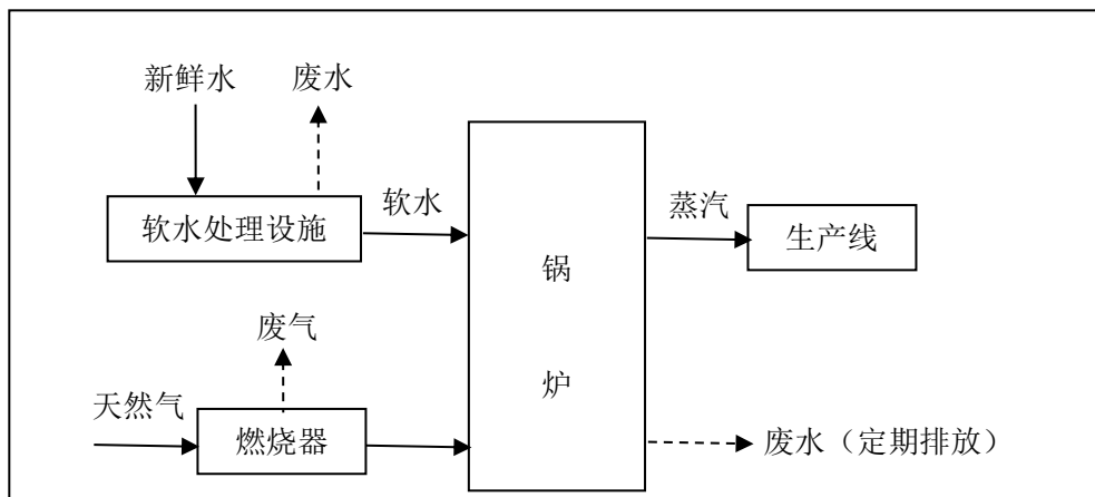
图2.8-1 锅炉运行流程图
