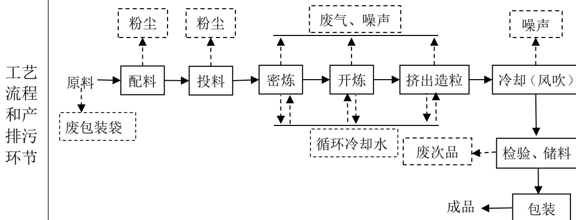
图 2-2 EVA 塑胶粒生产工艺流程及产污环节示意图
