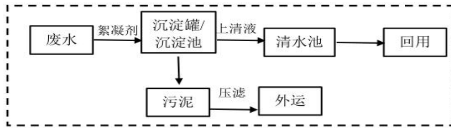
图 4-1 生产废水处理工艺流程图
