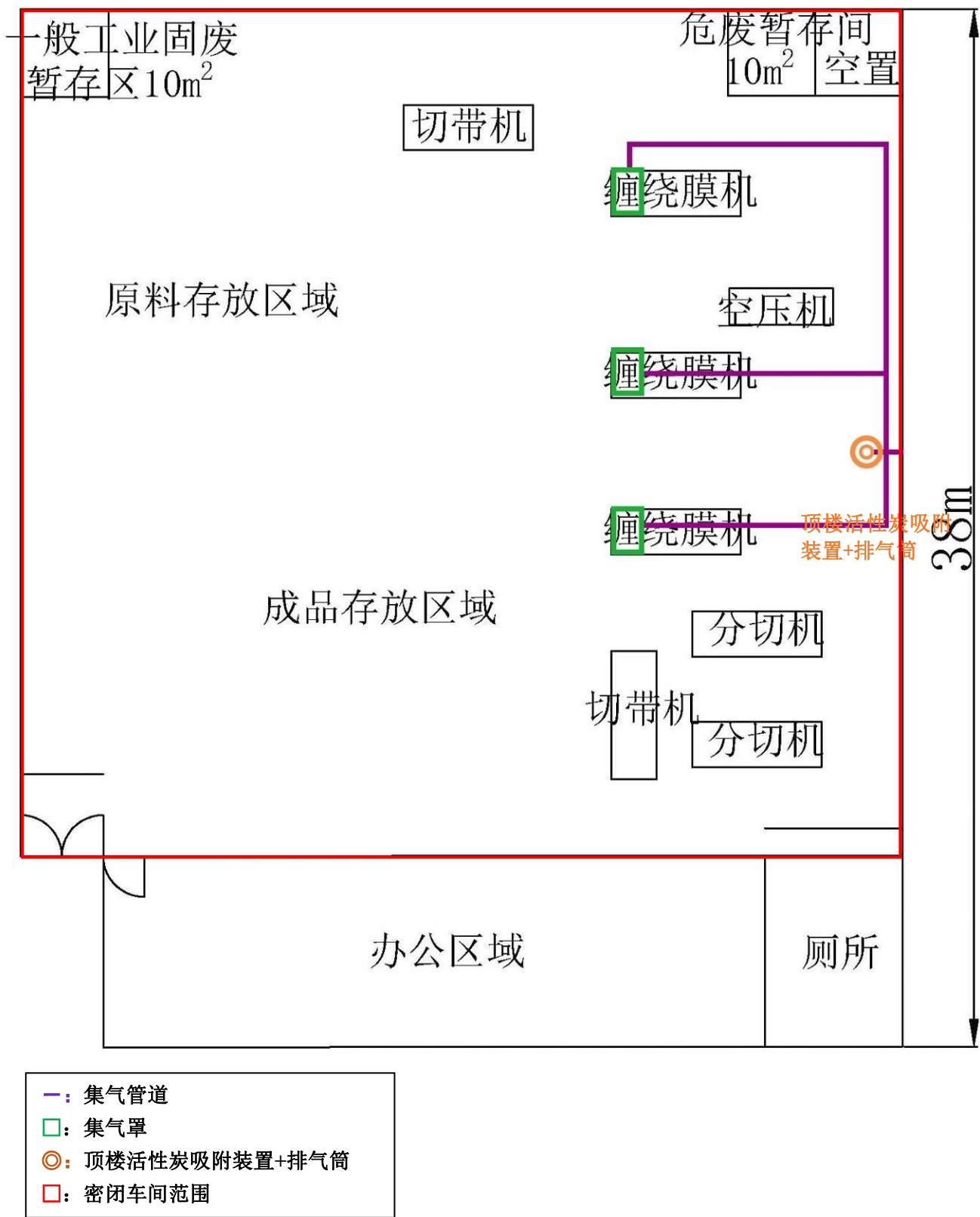
附图 1 本项目总平面布置图
