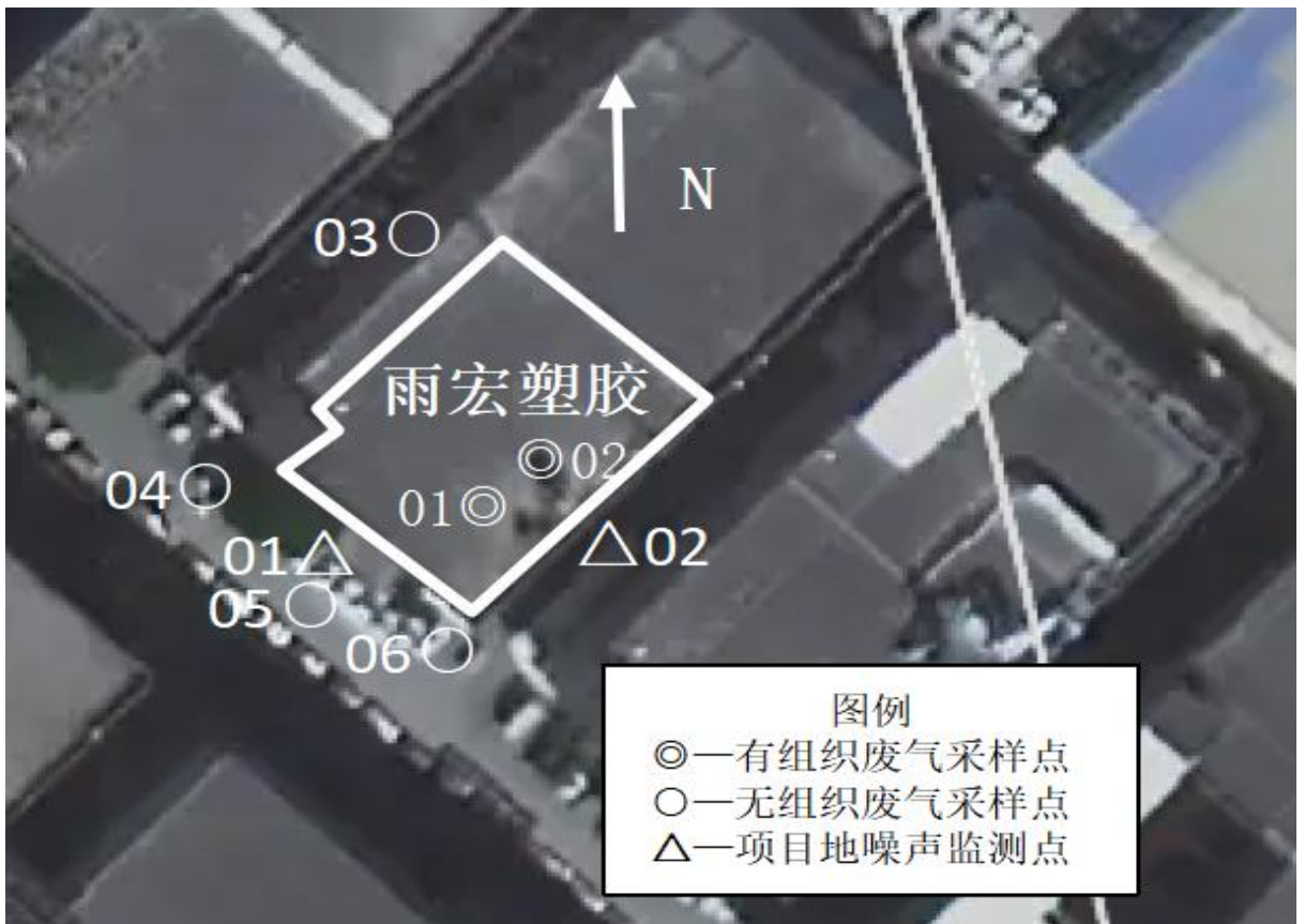
图 8-1 本项目竣工环境保护验收监测点位示意图
