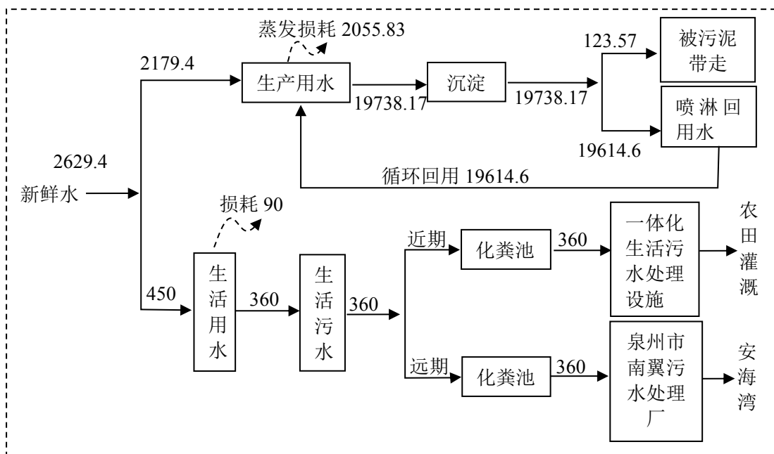
图 2-2 扩建后项目水平衡图（单位：m 3 /a）
