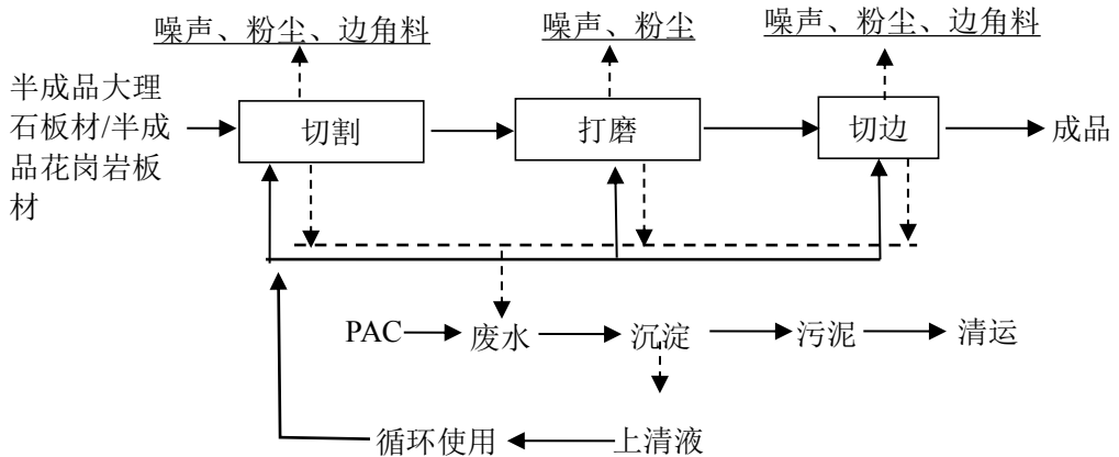
图 2-4 扩建前项目异形线条生产工艺流程图
