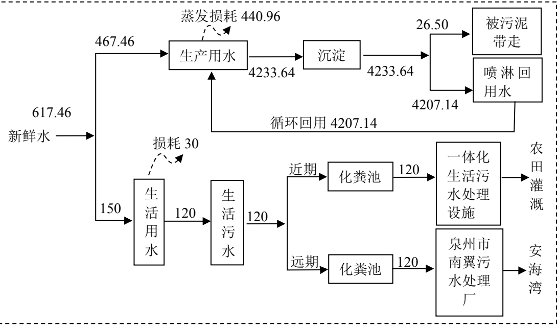
图 2-1 扩建项目水平衡图（单位：m 3 /a）
