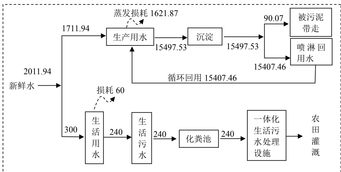
图 2-5 扩建前项目水平衡图（单位：m 3 /d）
