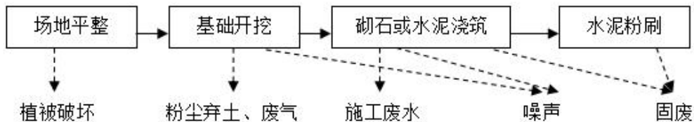
图 2.4-1 主体工程施工工艺流程及产污环节图
