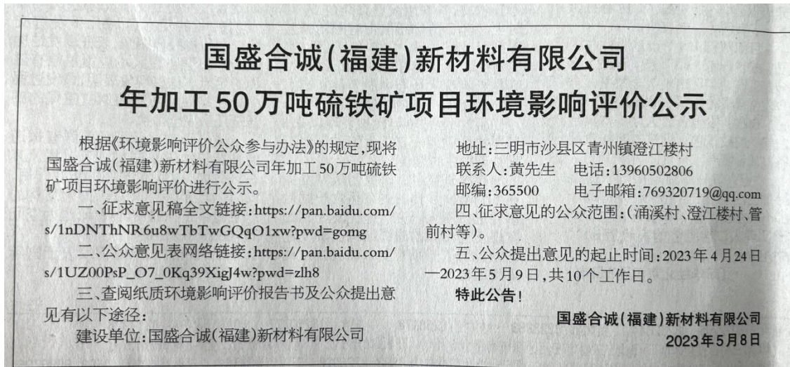
图3.2-2 项目环境影响报告书征求意见稿报纸公示照片
