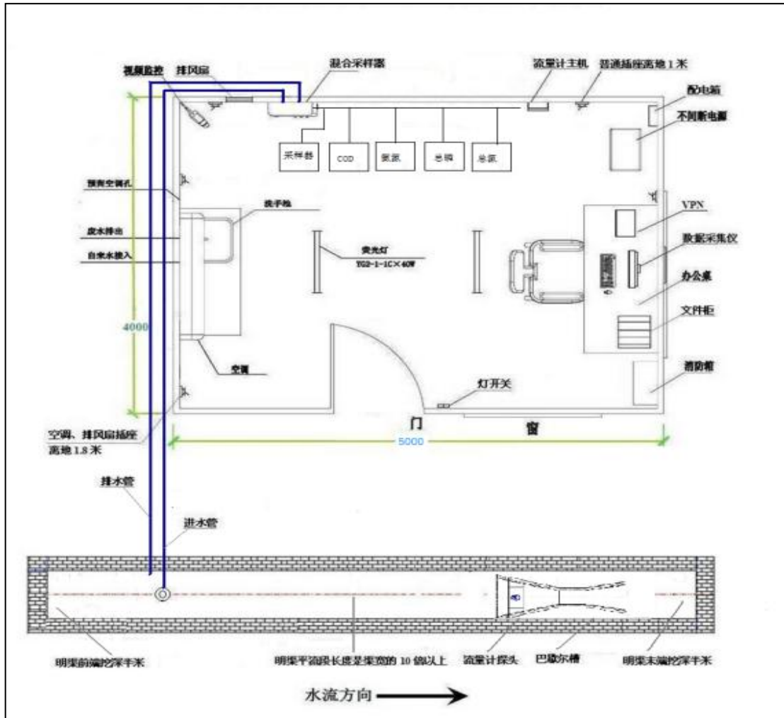
图 6.3 标准化排放口及在线监测房建设示意图
