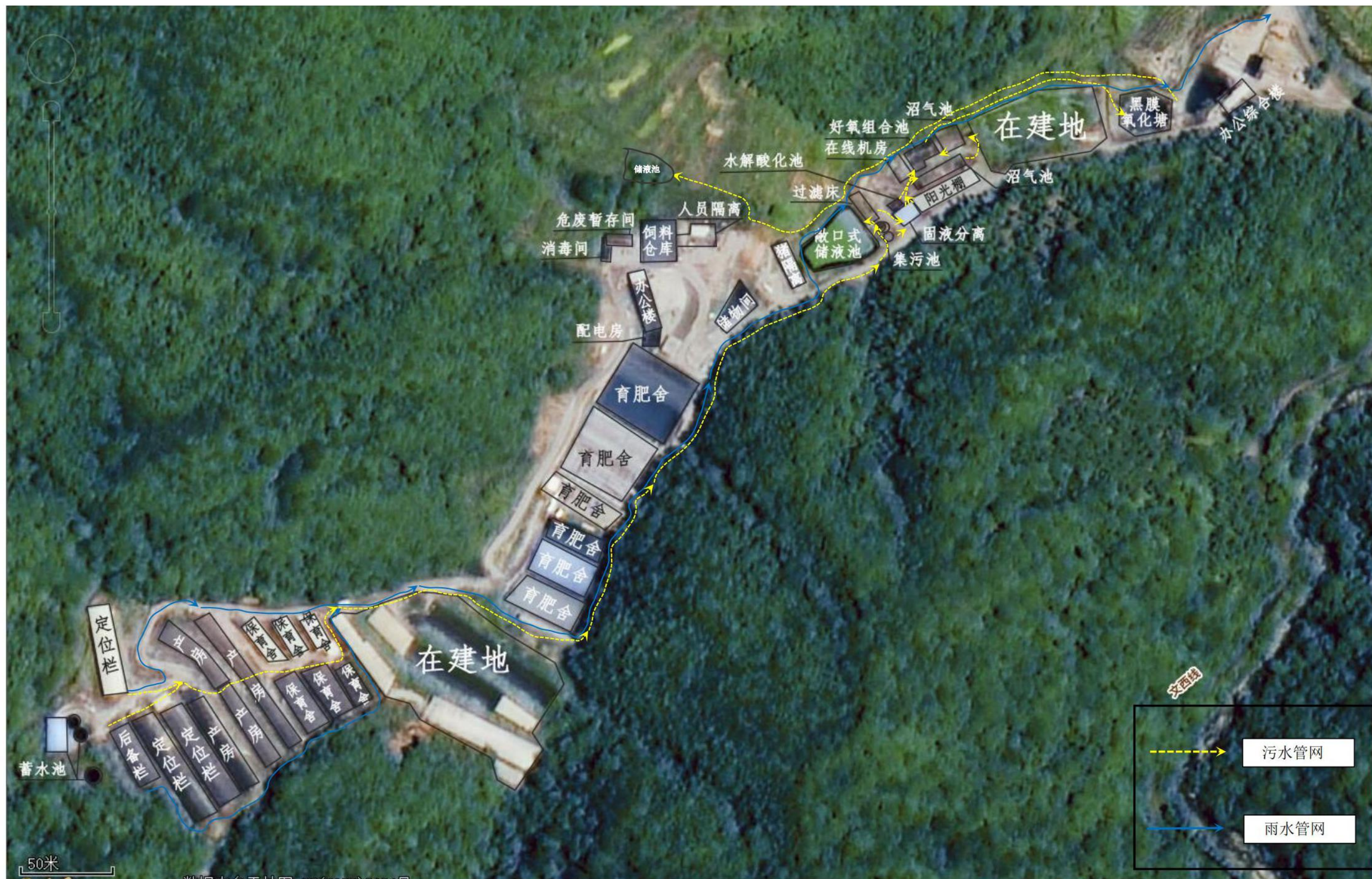
图 3.1-1 厂区平面布置图
