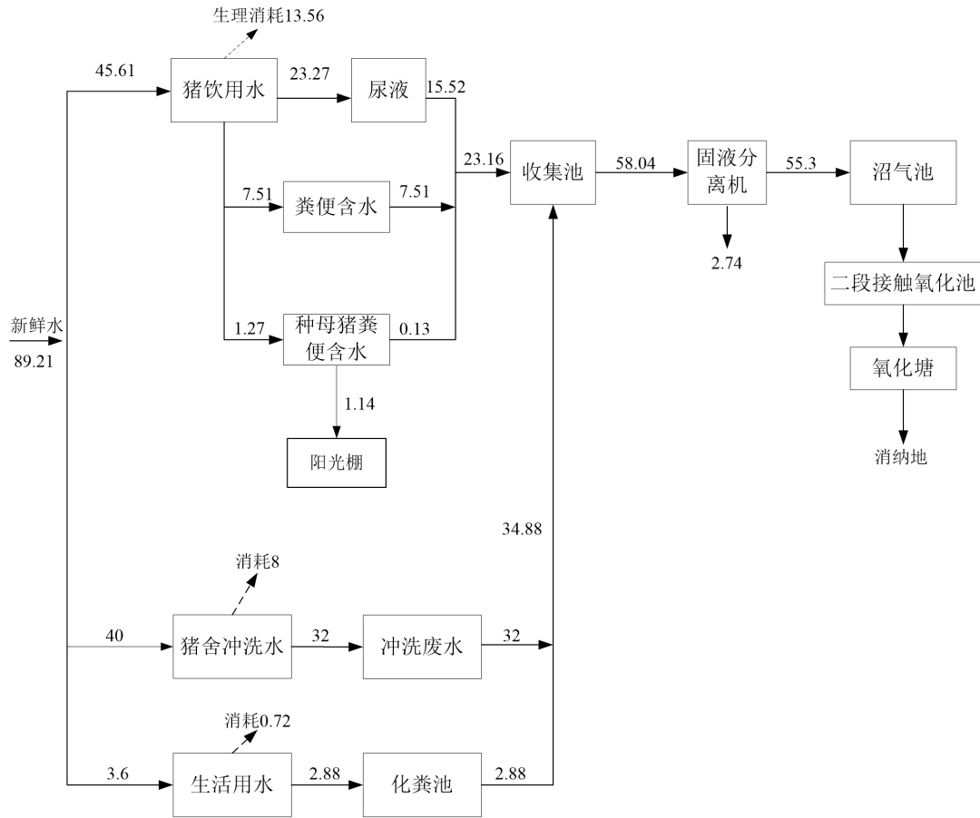
图 3.2-2 夏季全场水平衡图 (单位: t/d)
