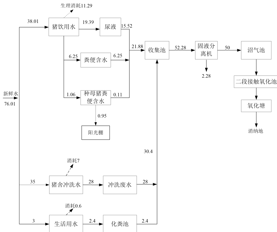
图 3.2-3 春、秋季全场水平衡图（单位：t/d）
