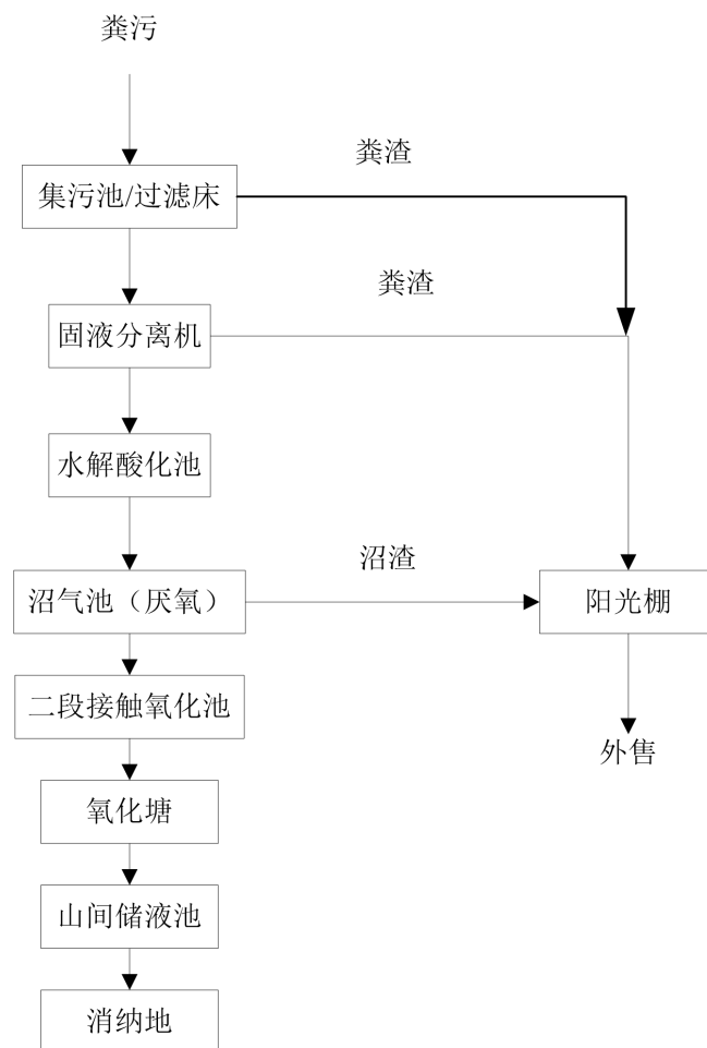
图 3.2-5 污水处理工艺流程图
