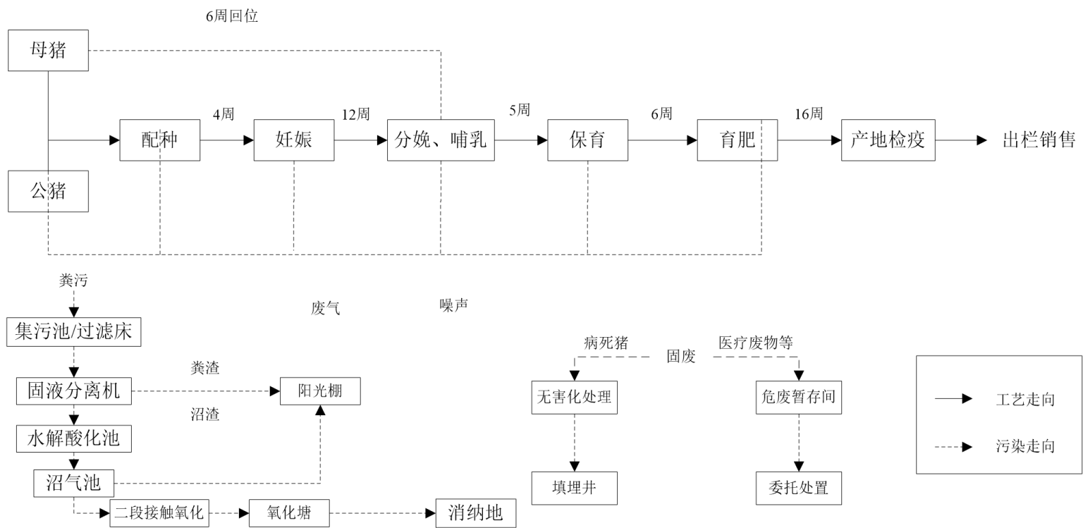
图 3.1-6 项目整体生产工艺流程
