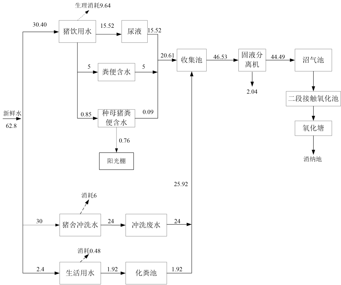
图 3.2-1 冬季全场水平衡图 (单位: t/d)
