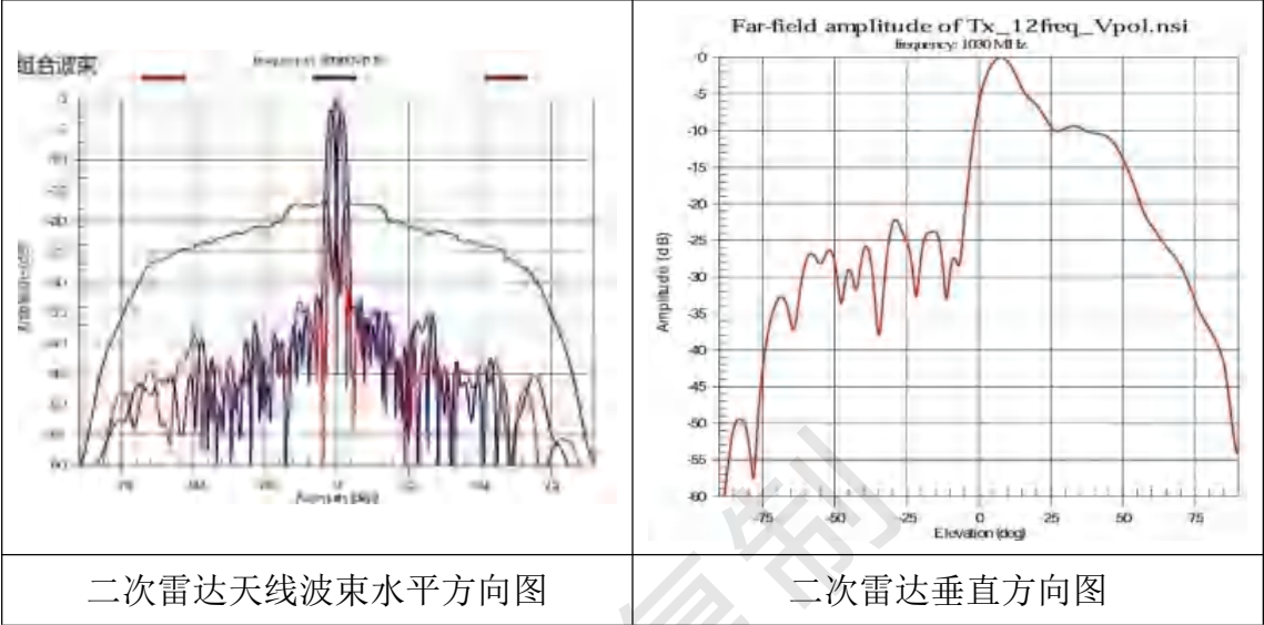
图 4.2-2 二次雷达水平、垂直方向图
