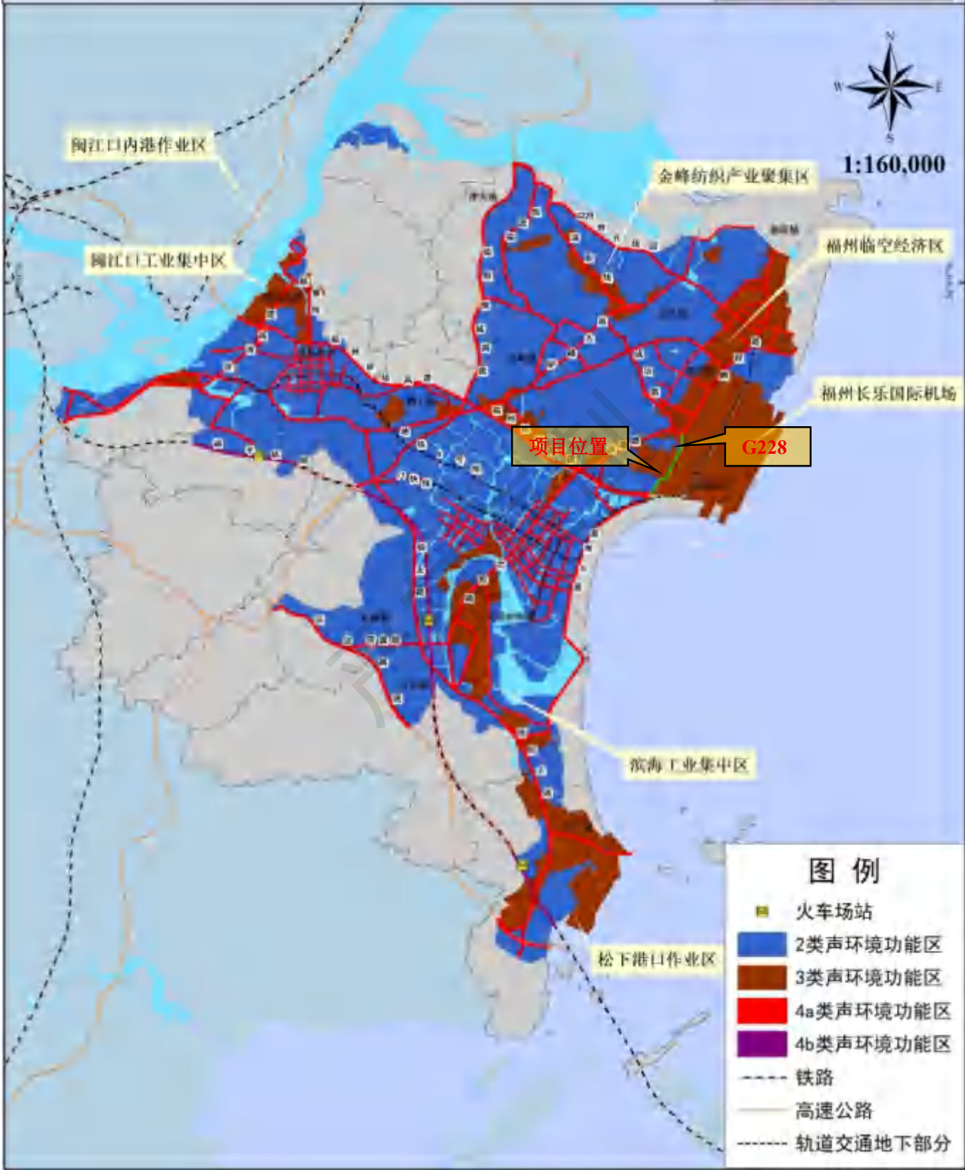
图 2.3-1 福州市长乐区声环境功能区划图
