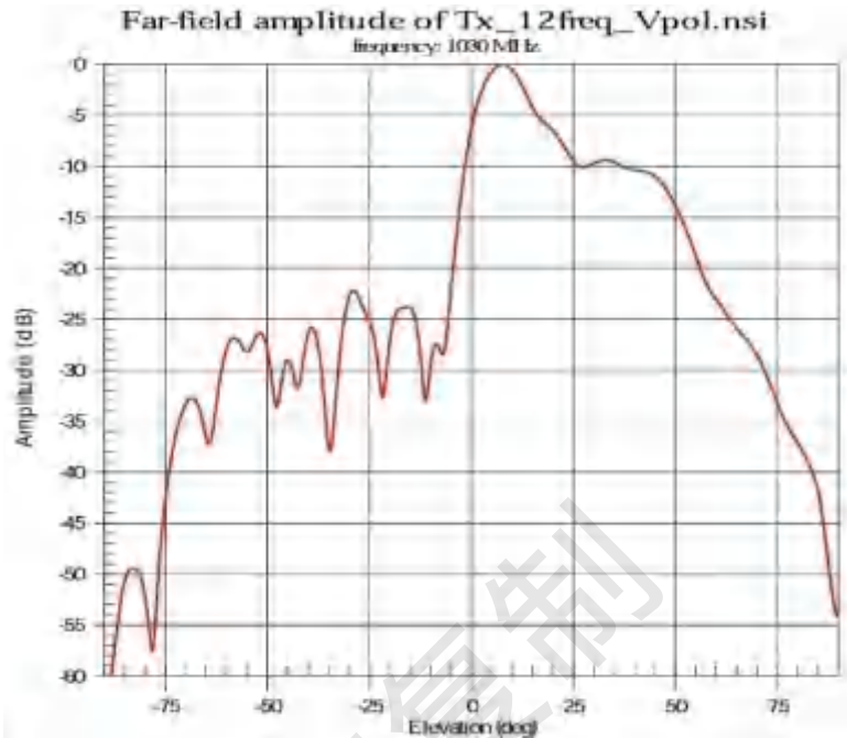
图 6.2-2 雷达天线垂直方向示意图
