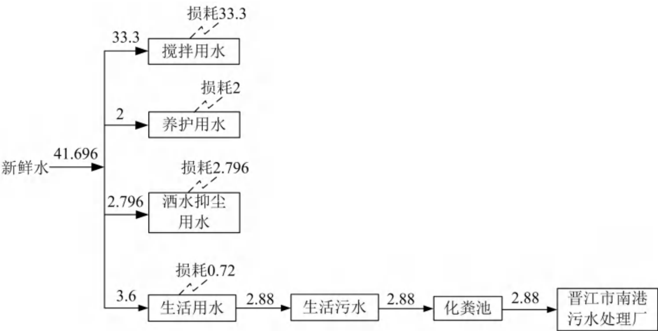
图 2-1 项目水平衡图 (t/d)
