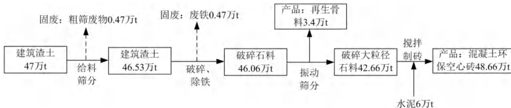
图 2-1 项目物料平衡图 (t/a)
