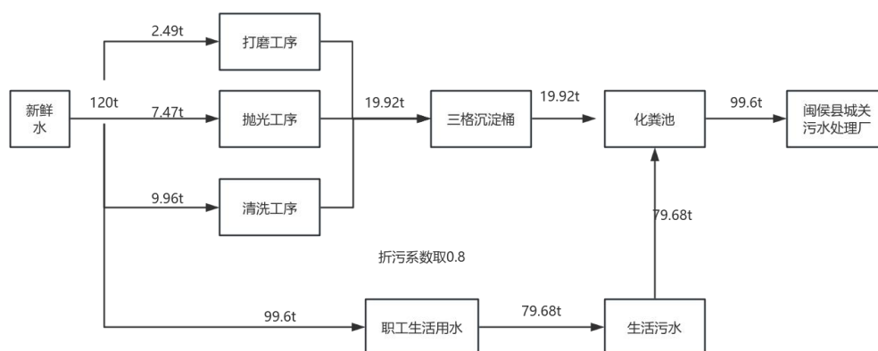
图 2.1-1 项目水平衡图（t/a）
