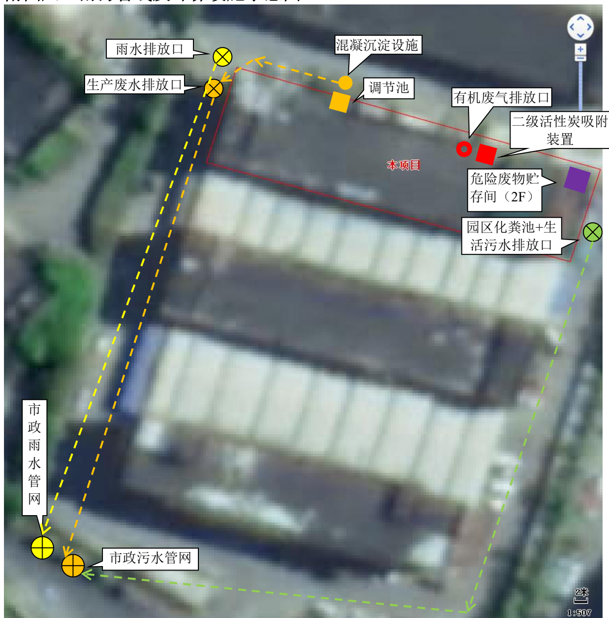
附图六：雨污管线及环保设施示意图
