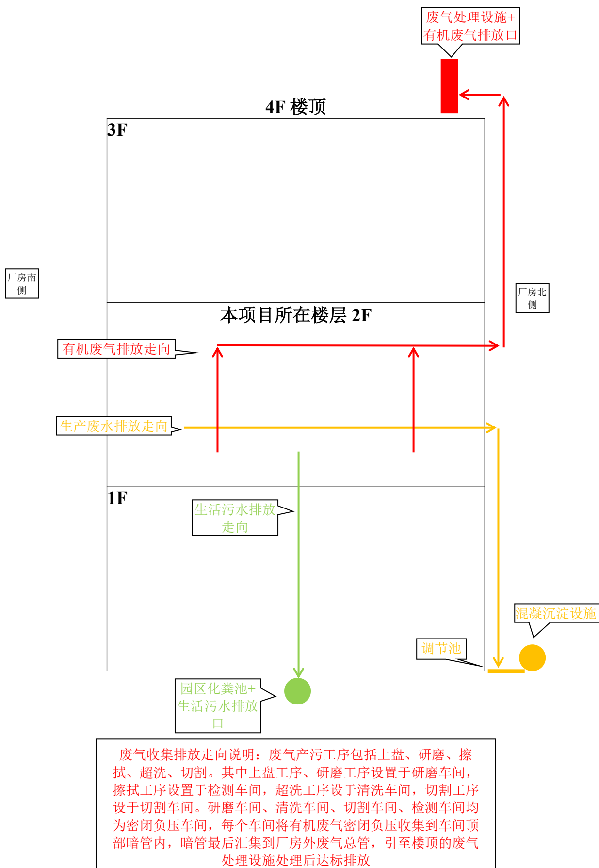
项目废水废气走向图（厂房右视图）
