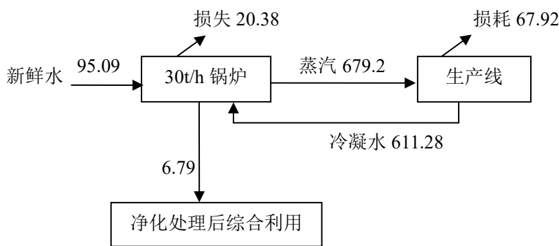
图 2.1-1 项目 30t/h 锅炉运行水平衡图 单位：t/d
